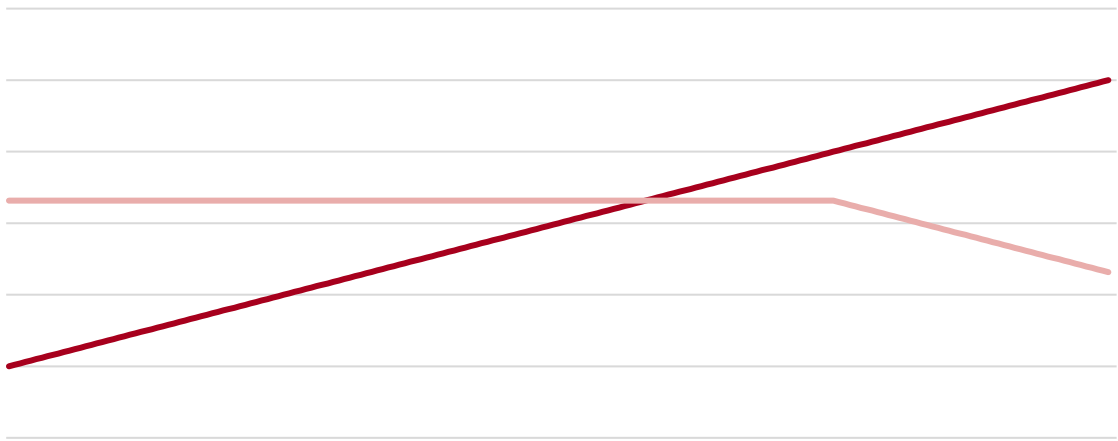
图表 11：备兑组合收益结构
